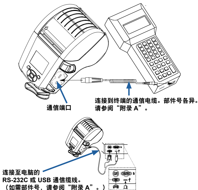
图 21 • 通信选项
