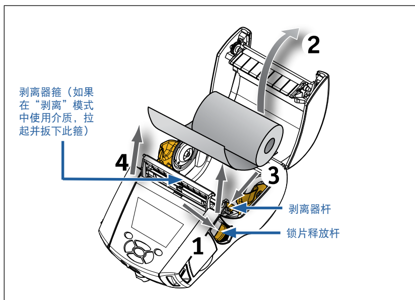
图 12 • 激活剥离杆（以 ZR668 Plus 为例）
