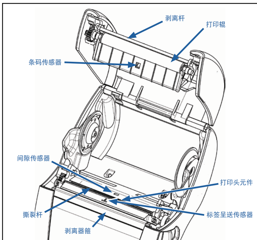
图 34 • ZR668 Plus 清洁 (带背衬)
