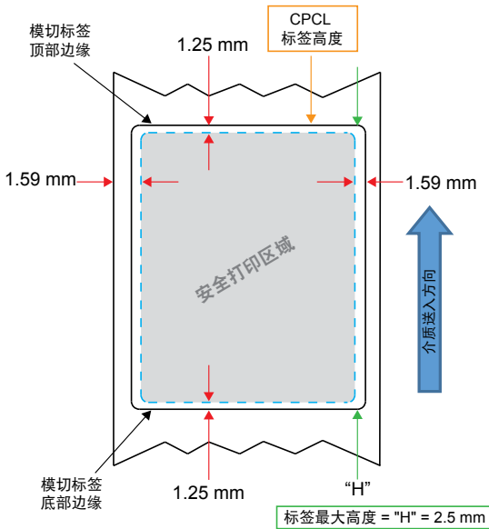
图 23 • 间隙介质
