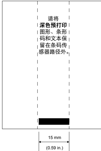
图 26 • 标签区域
