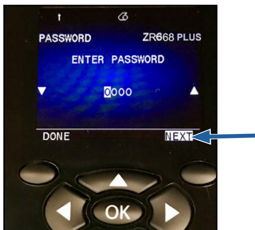
图 18 • 滚动菜单
