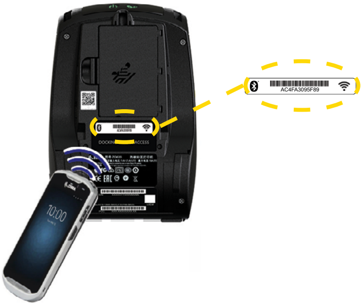
图 22 • 蓝牙/无线局域网通信
