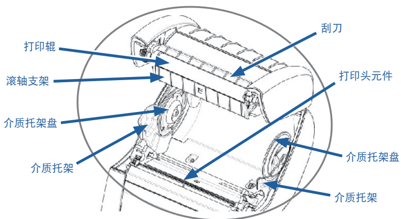
图 35 • ZR668 Plus 清洁 (无背衬)
