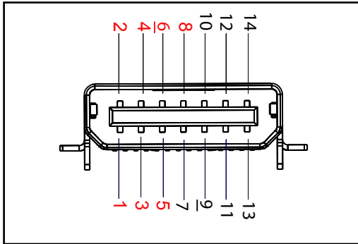
图 37 • RS-232C 通信端口
