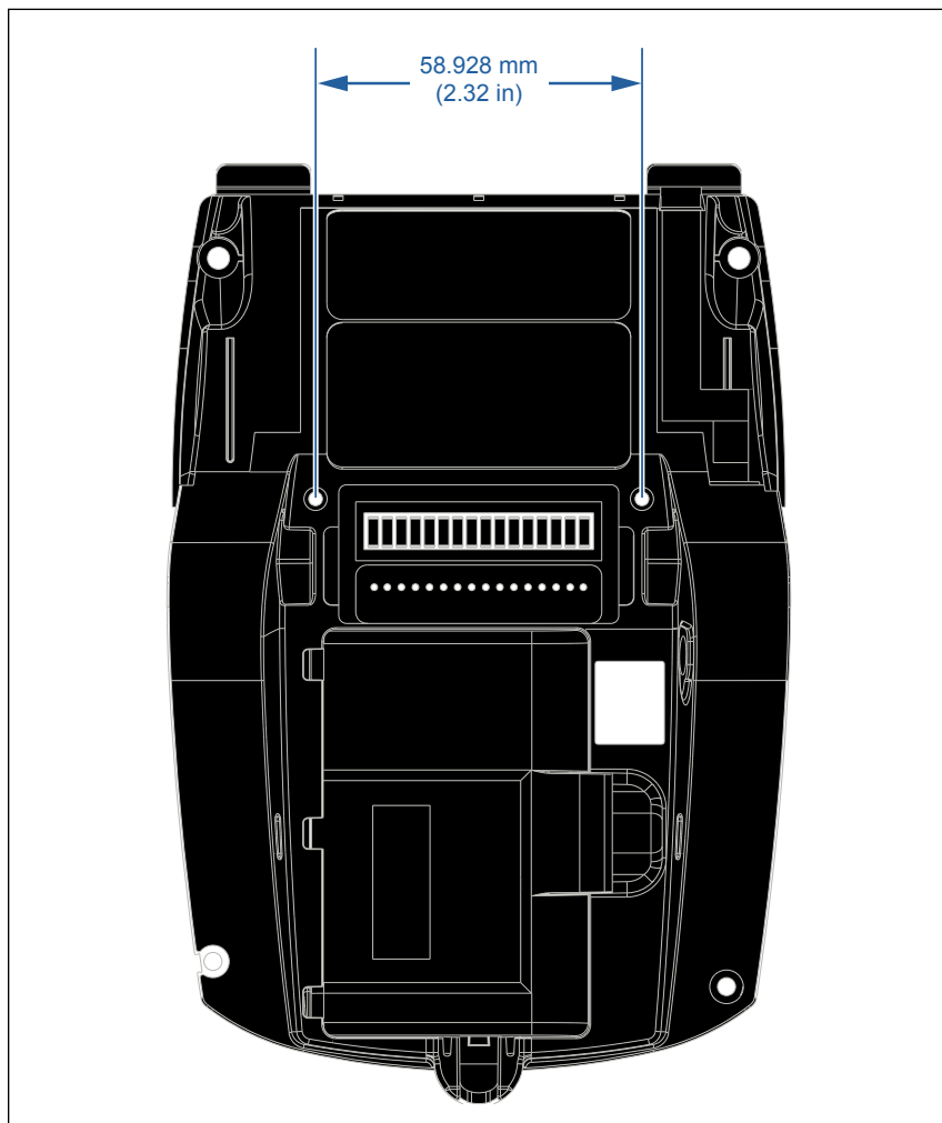
图 40 • ZR668 Plus 安装孔尺寸
