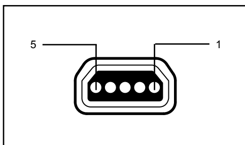
图 38 • USB 通信端口
