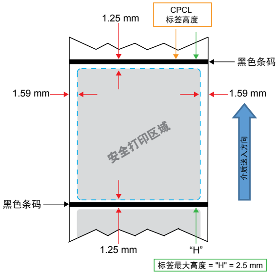
图 25 • 黑色条码标签介质
