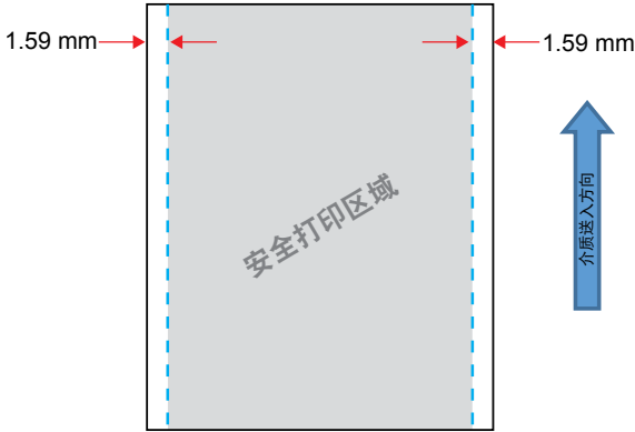
图 24 • 连续介质
