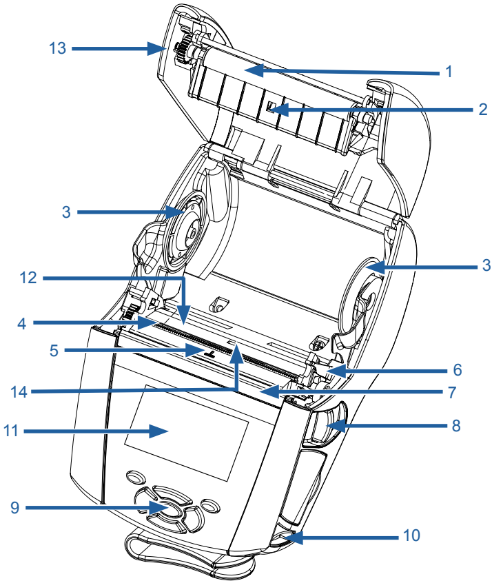
图 2 • 功能概览（图示为 ZR668 Plus）。
